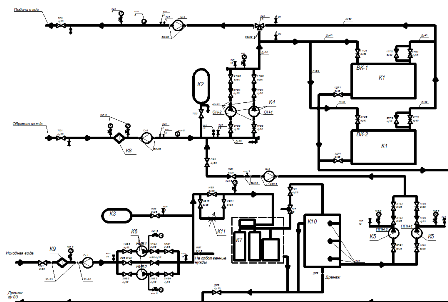
Рисунок 2.1 Схема отпуска тепловой энергии ТКУ-0,2 с. Богатое
