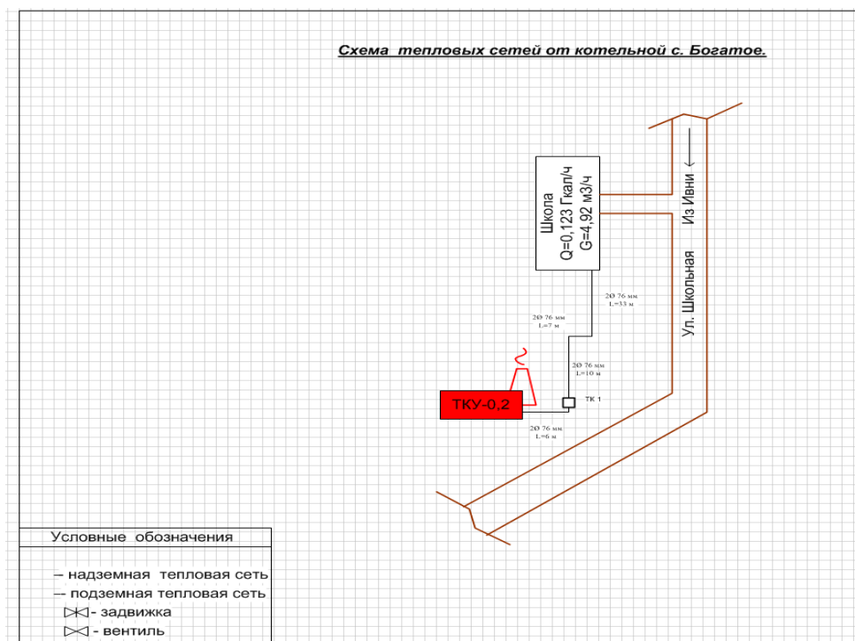
Рисунок 2 Схема тепловых сетей от котельной с.Богатое
