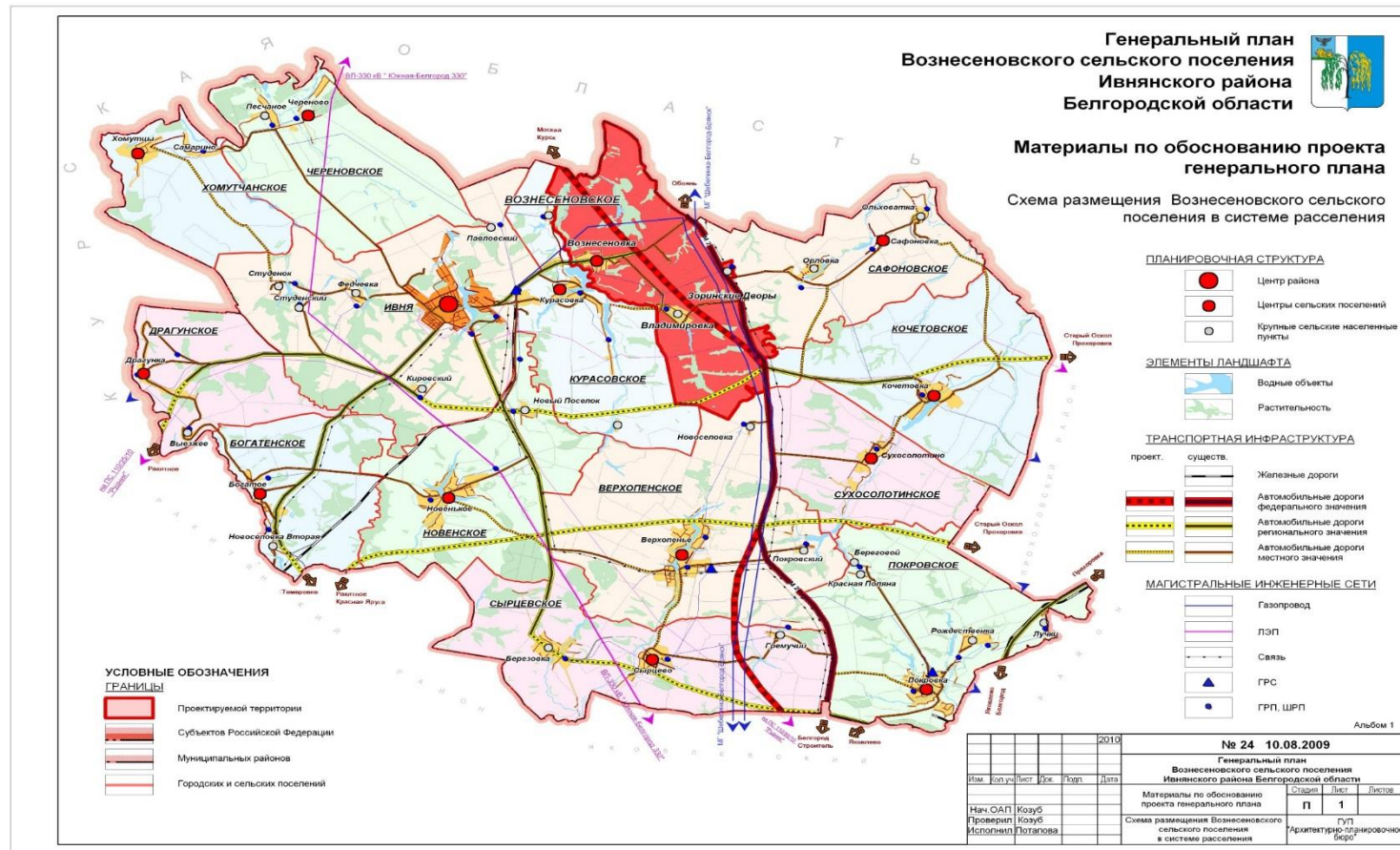
Рисунок 2. Зона действия ТКУ-0,2 Вознесенского сельского поселения
