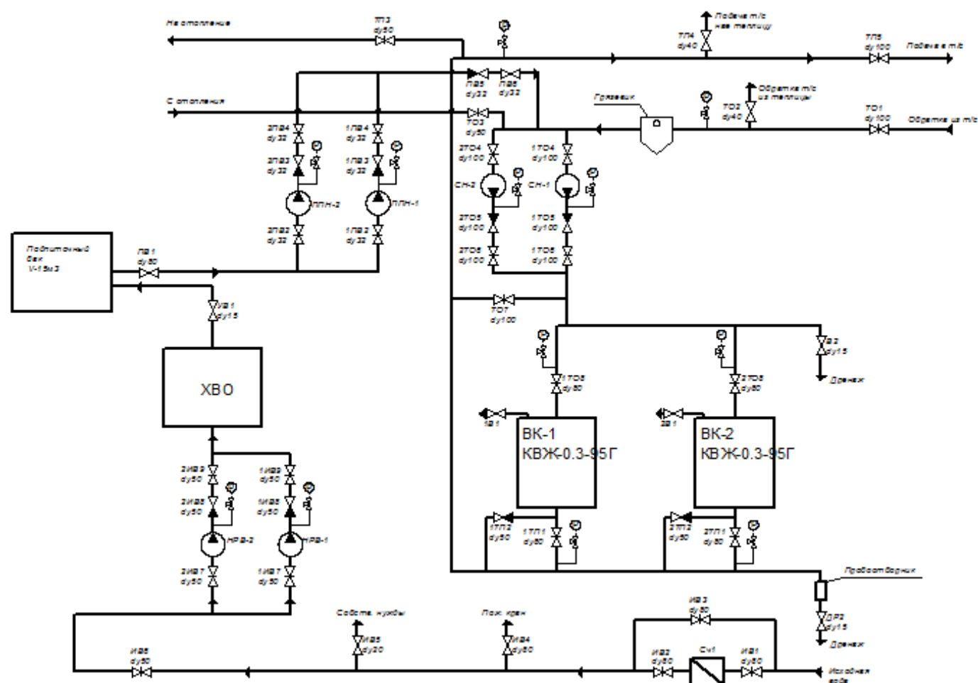
Рис. 3.1 Схема отпуска тепловой энергии котельной с. Владимировка
