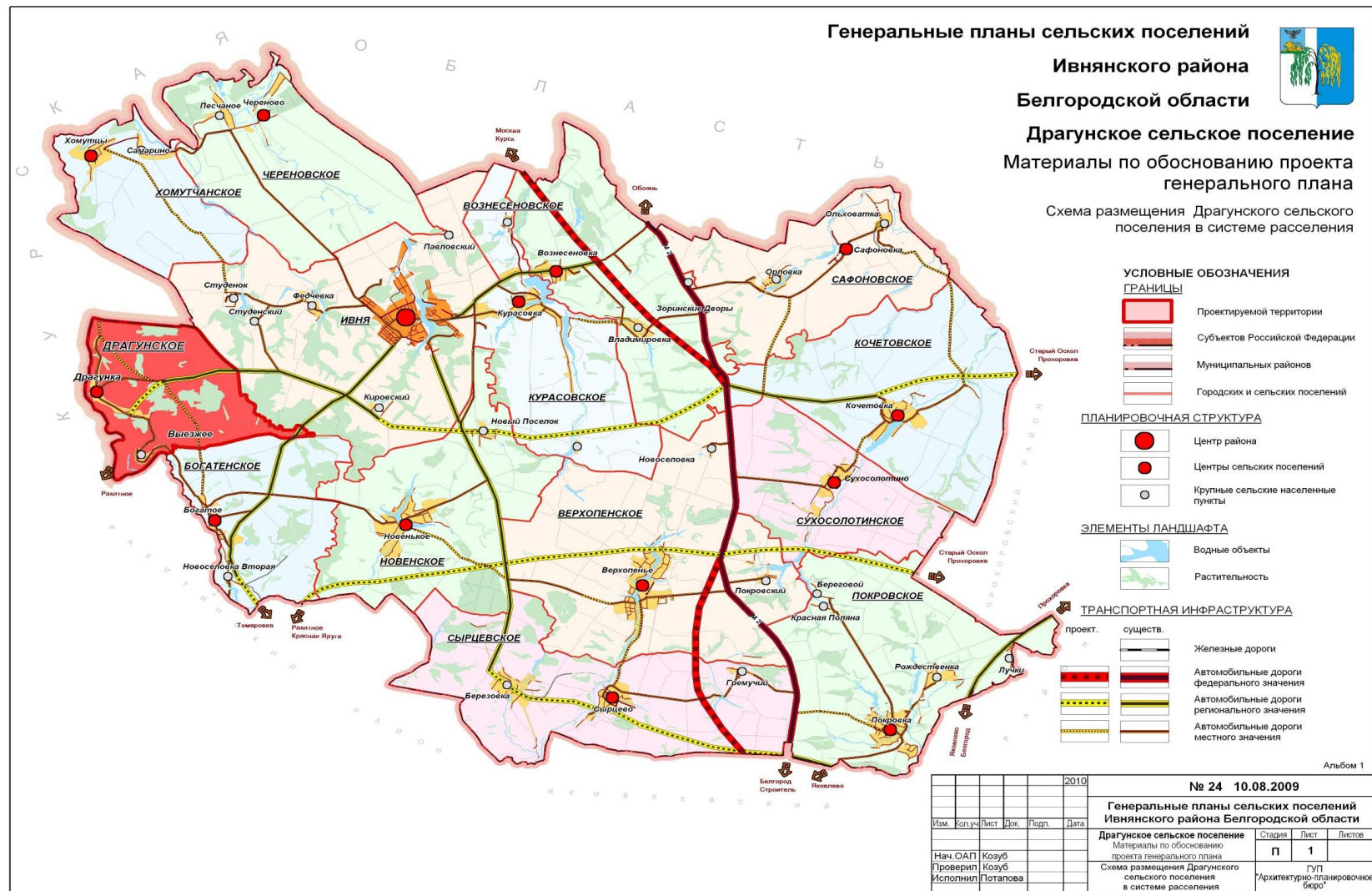
Рисунок 1. Зона действия котельной установки Драгунского сельского поселения
