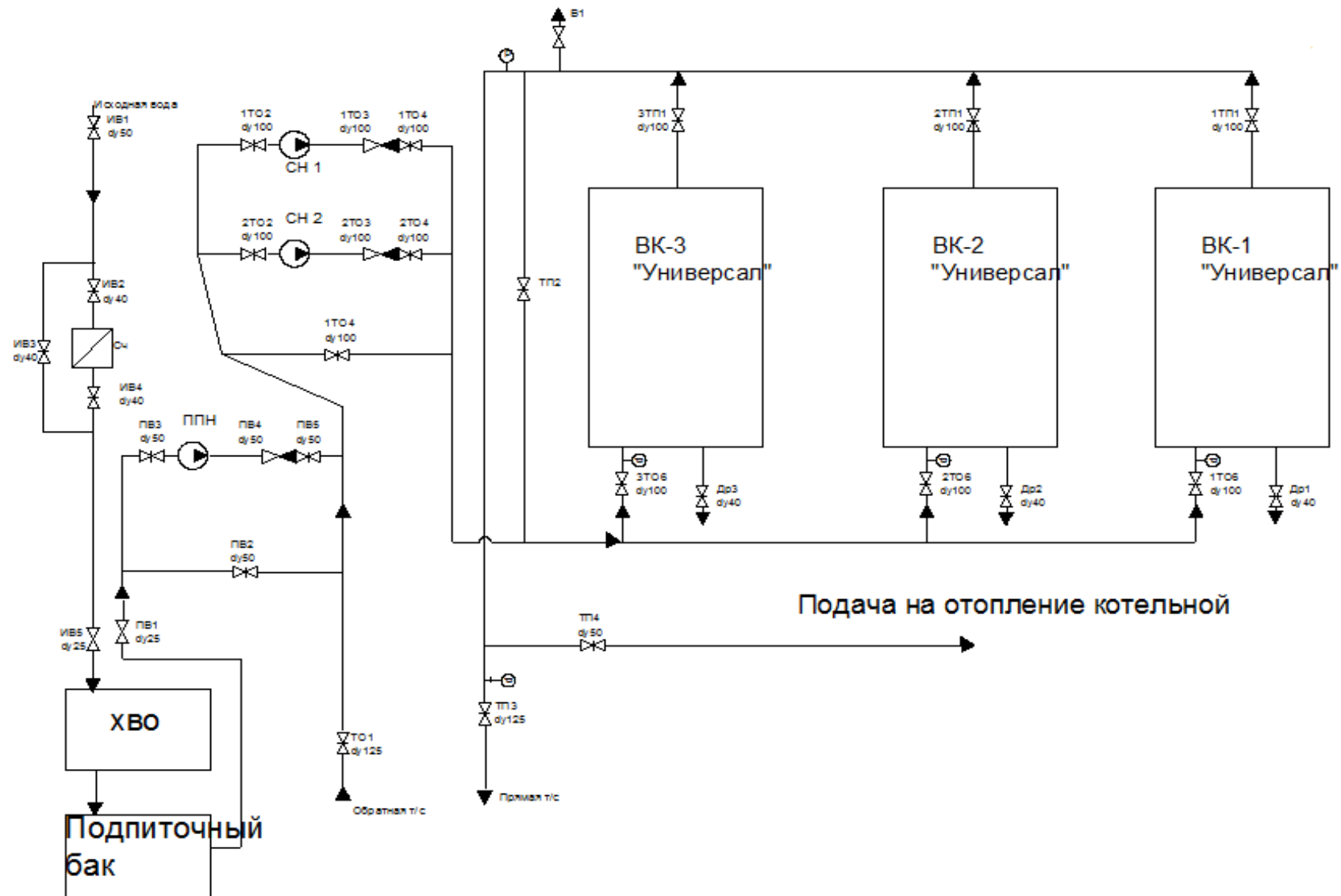
Рисунок 3. Схема отпуски тепловой энергии котельной с. Кочетовка
