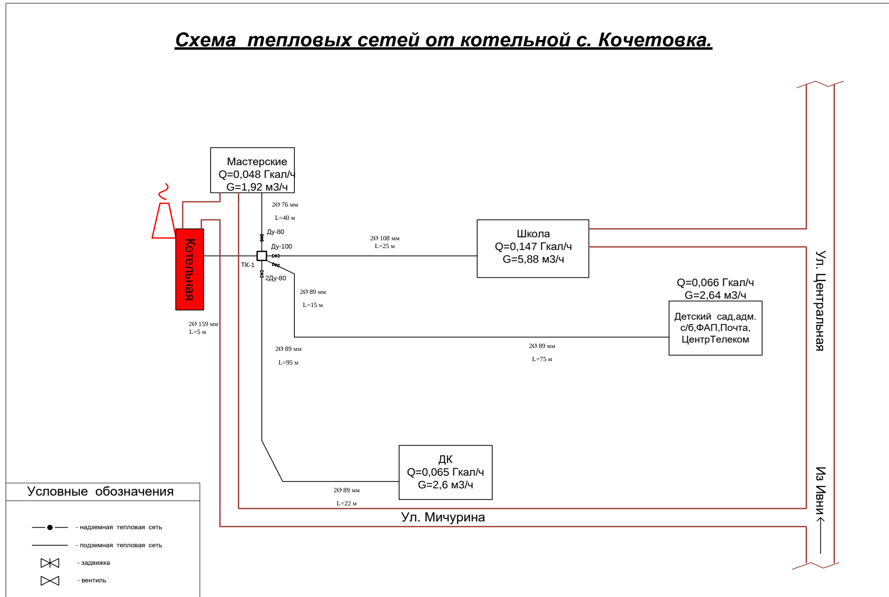
Рисунок 2. Схема тепловых сетей котельной с.Кочетовка
