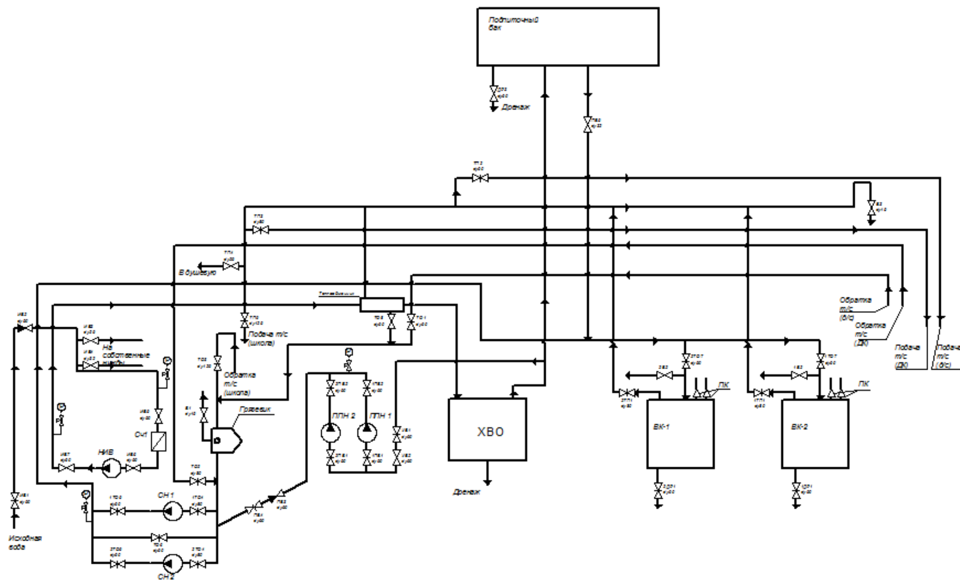
Рисунок 3. Схема отпуски тепловой энергии котельной с. Курасовка
