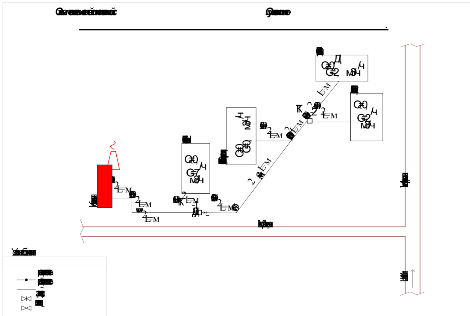
Рисунок 2. Схема тепловых сетей котельной с. Сухосолотино
