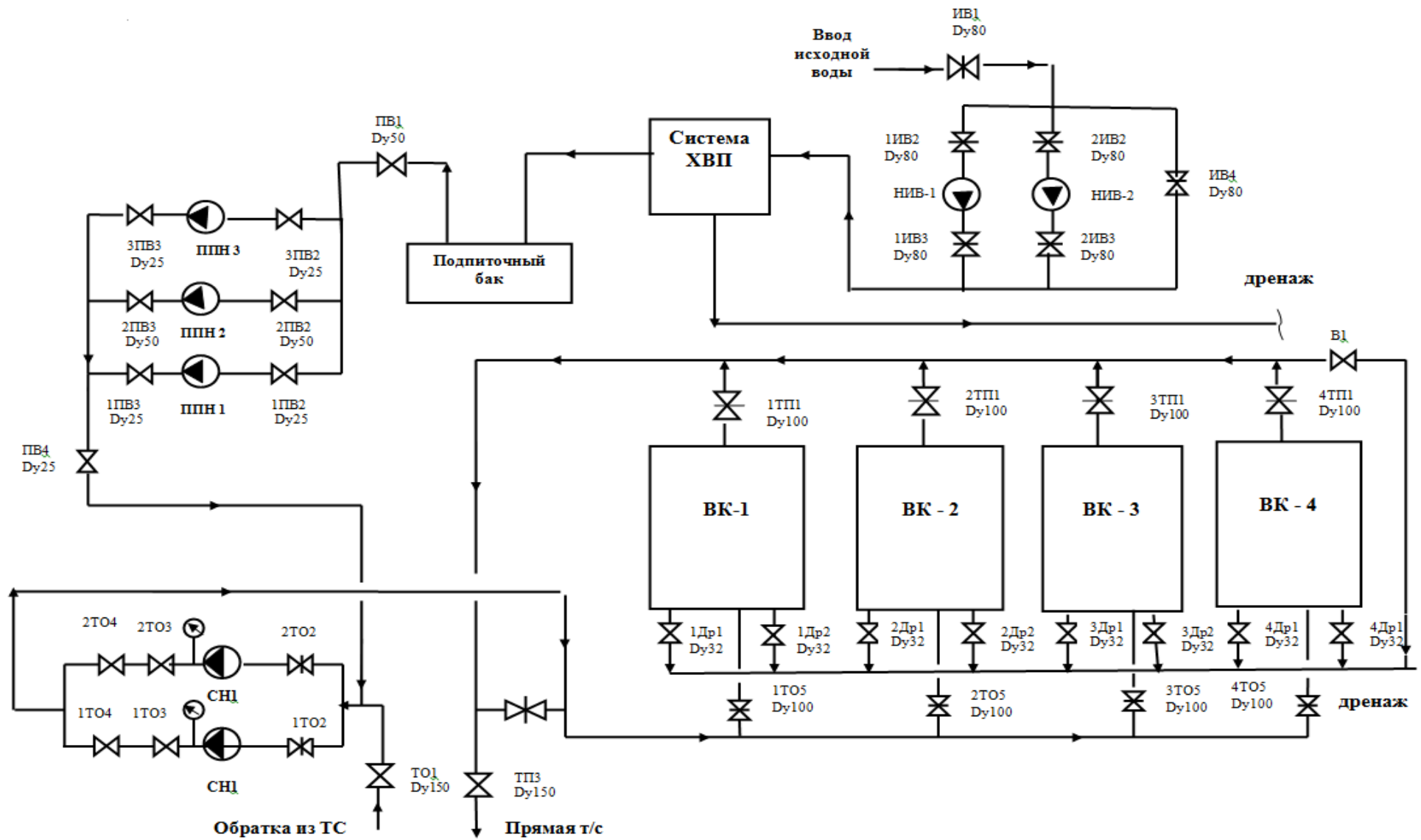
Рисунок 3. Схема отпуска тепловой энергии котельной с. Сырцево
